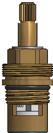
Cabeza Ceramica Vastago Medio
